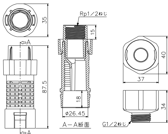
間接排水継手 EJK-20
