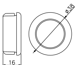
雨樋接続パッキン EJP-20
